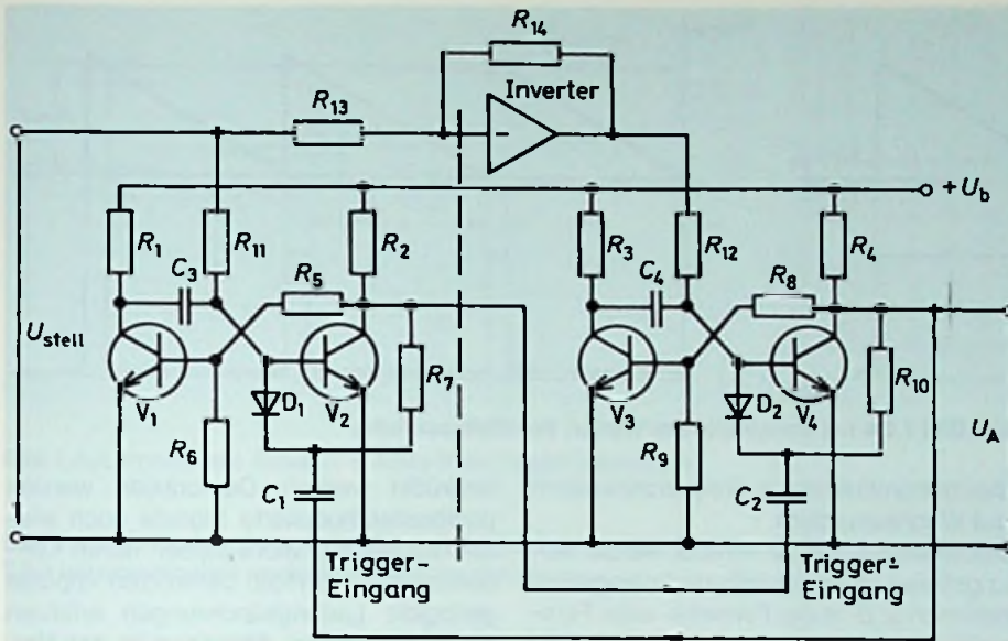
Bild 7.2.2: Monostabile Doppelkippstufe als Impulsbreiten-Modulator
