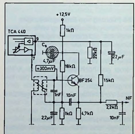
Bild 1: Schaltungsauszug des Demodulator-Teils
