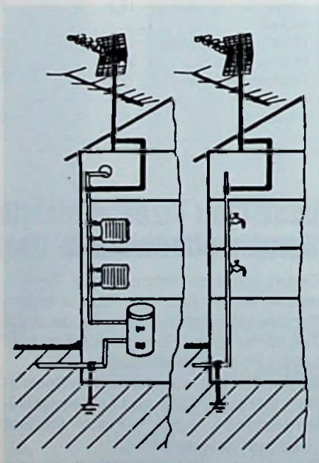
Bild 1: Durchgehend miteinander verbundene Wasser- oder Heizungsrohrleitungen aus Metall dürfen zur Erdung herangezogen werden
