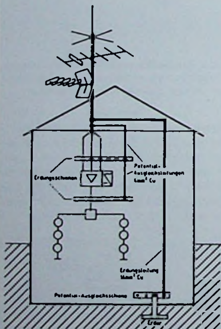
Bild 4: Beispiel für Erdungs- und Potentialausgleichsmaßnahmen bei einer GA-Anlage mit Dachantenne
