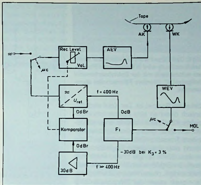
Bild 7: Automatischer MOL-Detektor
