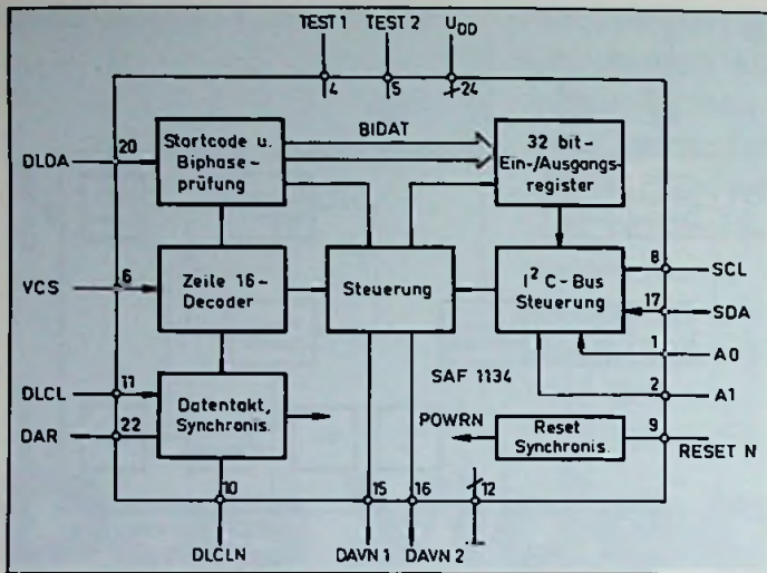
Bild 8: Blockschaubild des Datenzeilen-Decoders im integrierten CMOS-Baustein SAF 1134P (Bild: Valvo)
