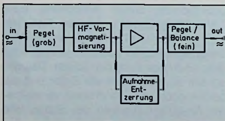
Bild 4: Blockschaltbild des RCLP-Systems
