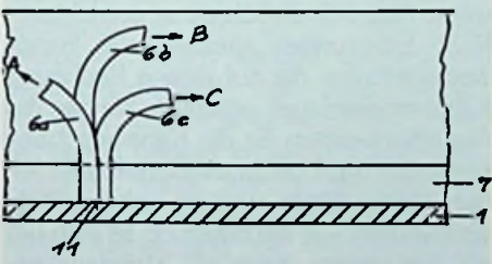
Bild 2: Schnitt durch den Flachbildschirm mit Lichtleitfasern
