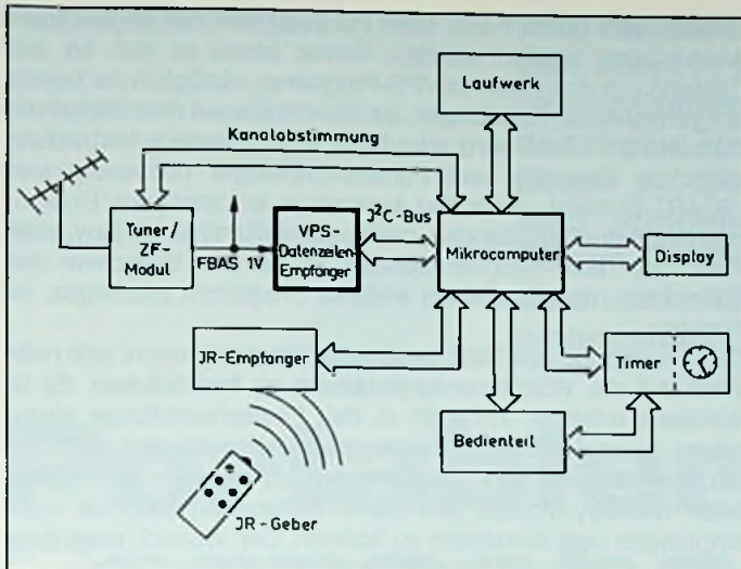
Bild 6: Vereinfachtes Blockschaltbild eines Videorecorders mit integriertem VPS-Datenzeilenempfänger
