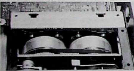
Bild 3: Im konstruktiven Aufbau des riemengekoppelten Doppel-Capstan sind die Statorspulen organisch in den Platinenaufbau der PLL-Steuerungselektronik einbezogen
