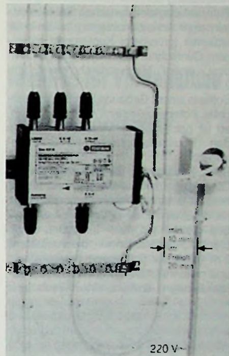
Bild 2: Beispiel für das richtige Einhalten des Abstandes zwischen einer spannungsführenden Leitung und einem Antennenkabel
