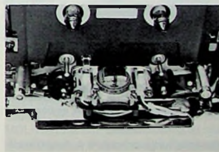
Bild 2: Der Vierspurkopf (Bildmitte) dreht sich bei Spurenwechsel um 180°
