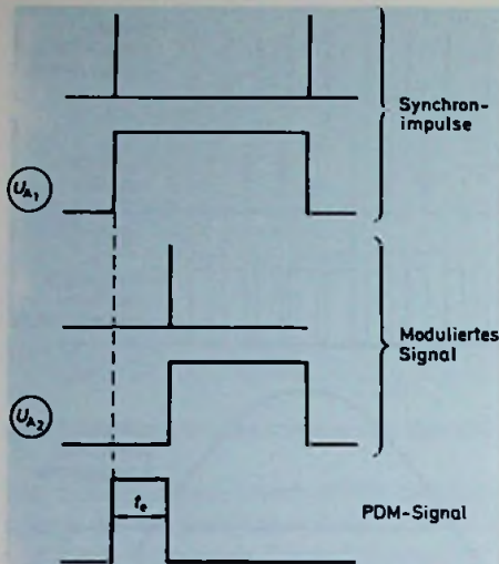
Bild 7.3.8: Zeitlicher Verlauf der Spannungen im Bild 7.3.7
