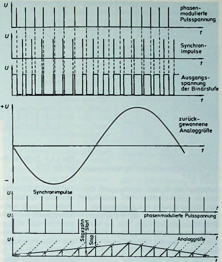
Bild 7.3.5: Spannungsverhältnisse bei einem Demodulator für phasendemodierte Pulsspannungen mit Sägezahn-generator
