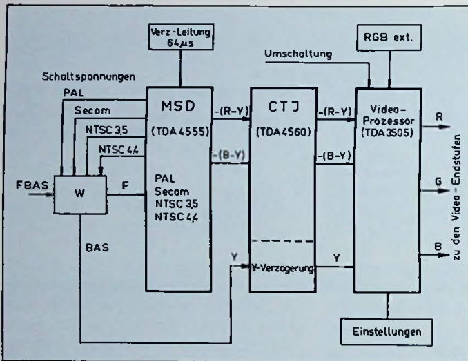
Bild 3: Die vereinfachte Blockschaltung des Multistandard-Farbdecoders mit CTI-Farbsprungversteigerung und nachfolgendem Video-Prozessor
