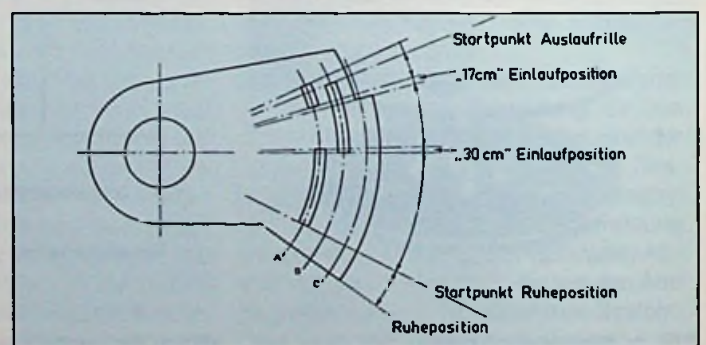
Bild 7b: Die Kodierplatte des 3-bit-Encoders
