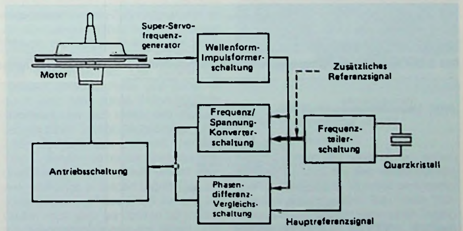
Bild 3: Blockschaltung der Doppelservo-Quarzsteuerung
