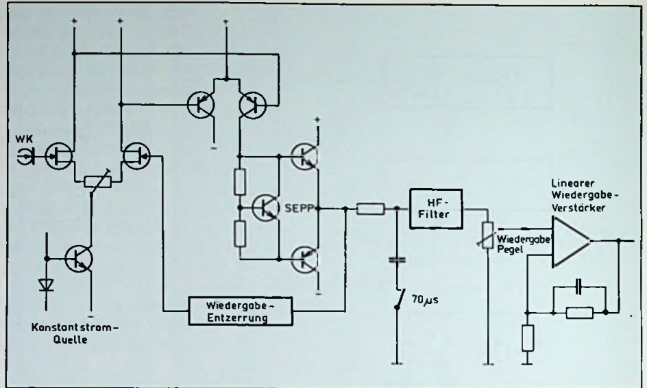
Bild 9: Die Eingangsstufe des Wiedergabe-Entzerrungsverstärkers
