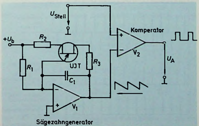
Bild 7.2.4: Sägezahngenerator und Komparator als Impulsbreiten-Modulator
