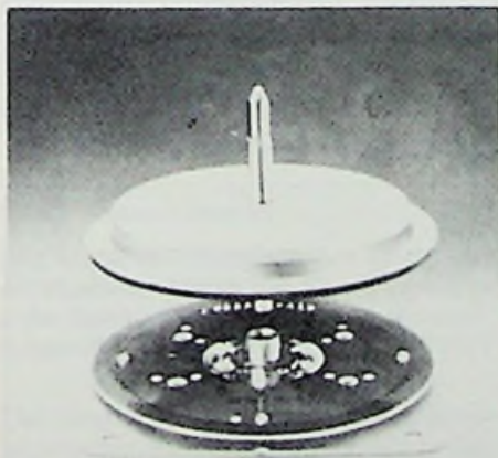
Bild 2: Direktantriebsmotor mit über den Statorspulen angeordneten Rotormagneten
