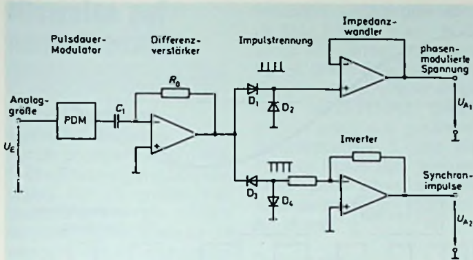
Bild 7.3.2: Prinzipielle Schaltung eines Pulsphasenmodulators
