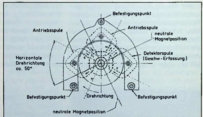
Bild 6: Der mechanische Aufbau des horizontalen Tonarmantriebes
