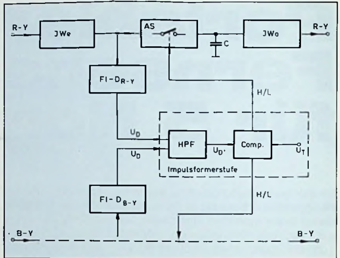
Bild 4: Das Funktionsschema der Versteigerungsschaltung in den Farbdifferenzkanälen durch das CTI-Verfahren (ohne Verzögerung im Leuchtdichtekanal)
