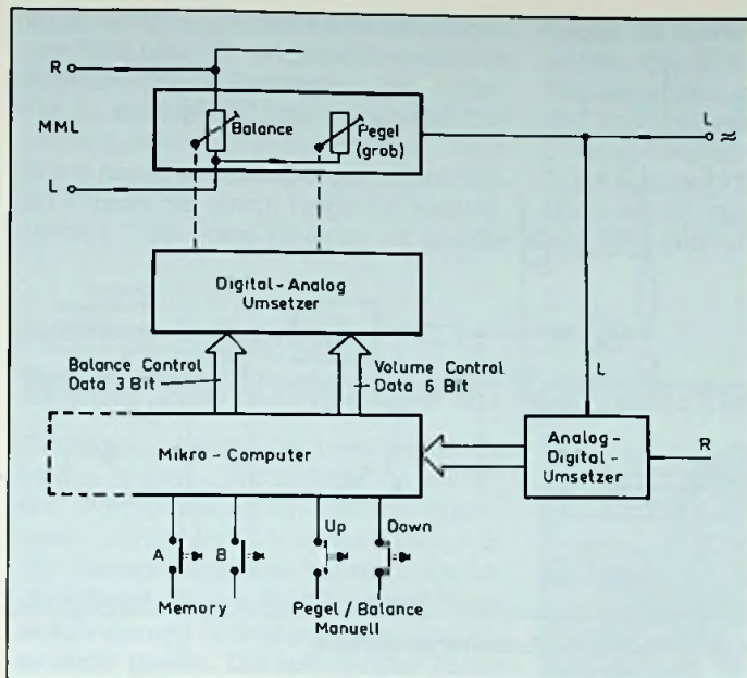
Bild 5: Pegel- (grob) und Balance-Einstellung in der ersten Funktionsstufe des RCLP-Systems
