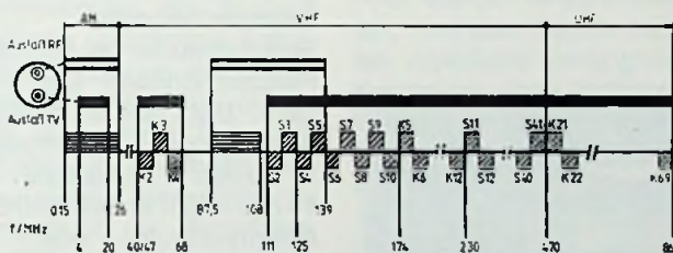
Bild 1: Frequenzbereiche, die über die neue Antennensteckdose übertragen werden können (Hirschmann-Presebild)
