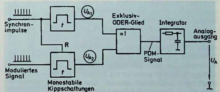
Bild 7.3.7: Möglichkeit der Pulsphasen-Demodulation mit Koinzidenz-Demodulator
