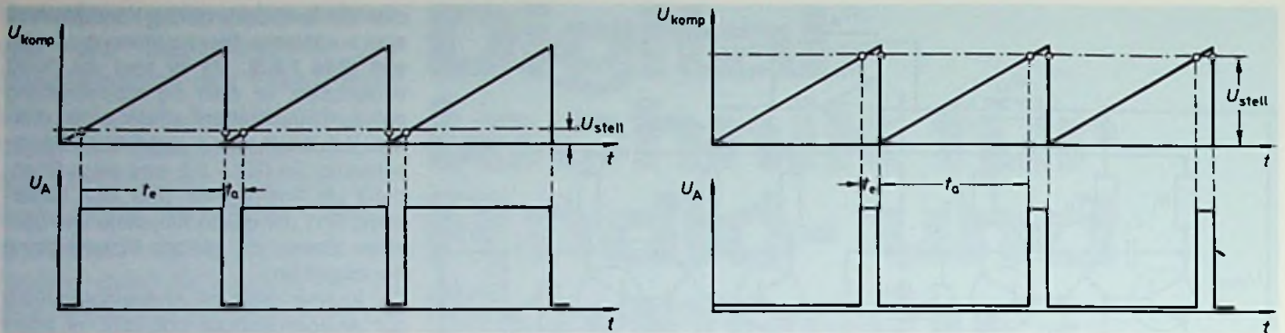
Bild 7.2.5: Ausgangsspannung des Komparators in Bild 7.2.4 bei verschiedenen Werten der Stells Spannung
