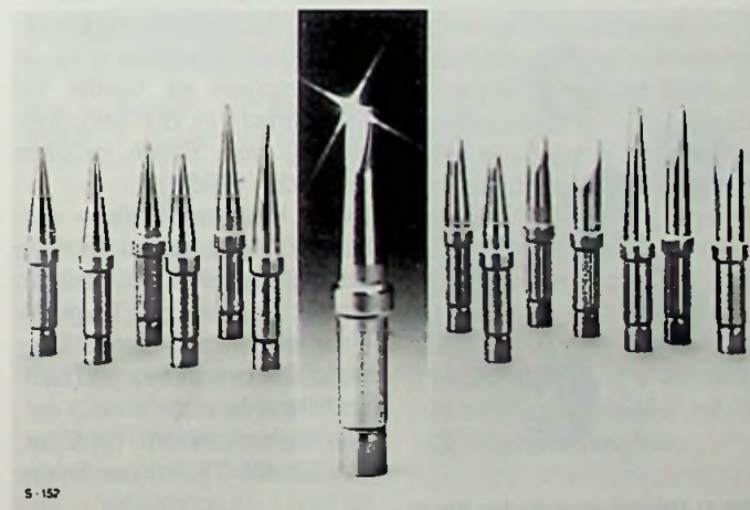
Bild 1: Lötpitzen mit neuartiger Oberflächenbeschichtung (Ernest Spirig-Pressebild)
