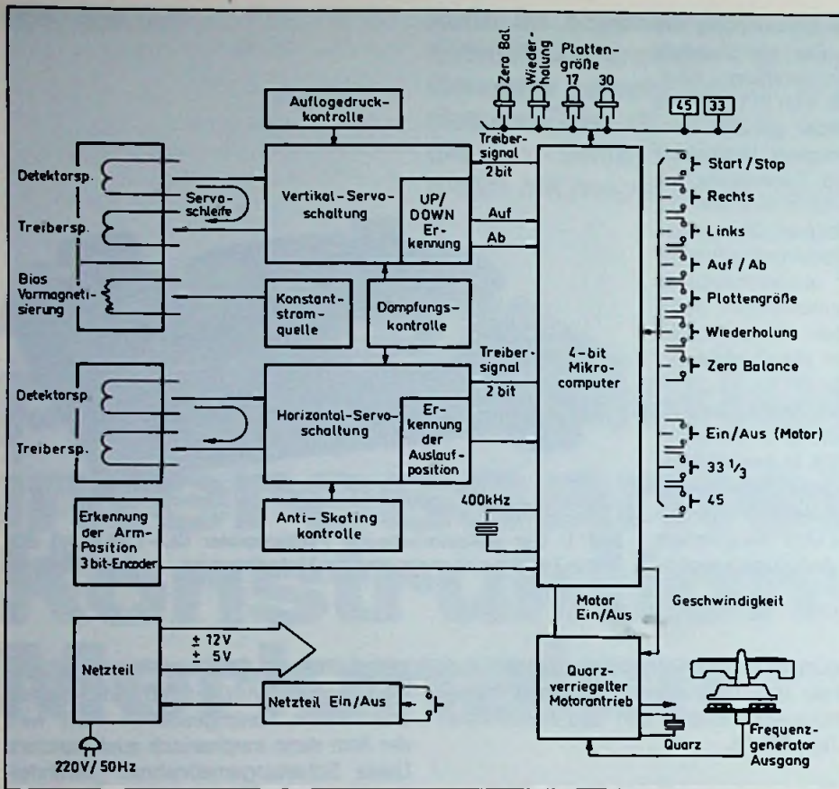
Bild 4: Blockschaltung des ED-Servo-Tonarms
