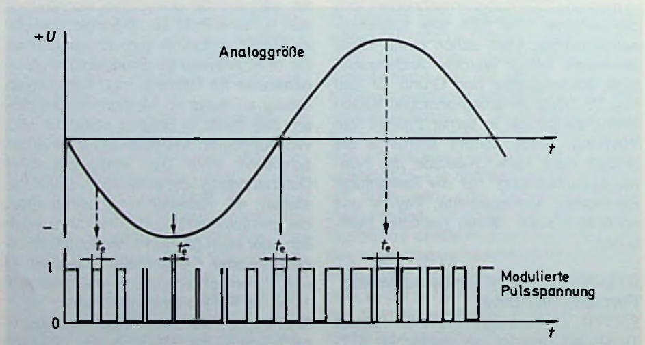
Bild 7.2.1: Abhängigkeit der Pulsdauer von der Analoggröße bei der PDM
