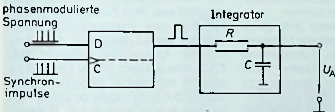
Bild 7.3.3: Demodulator für pulphasenmodulierte Signale mit Binärstufe
