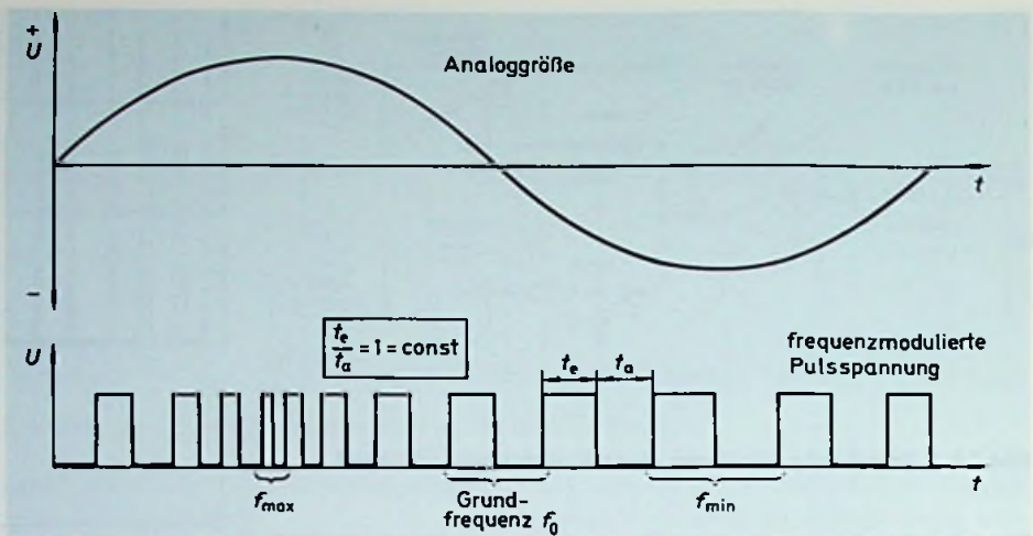
Bild 7.4.1: Zeitlicher Verlauf der Analogspannung und der dazugehörigen Pulsspannung bei der PFM
