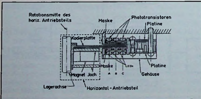
Bild 7a: So ist der 3-bit-Encoder aufgebaut
