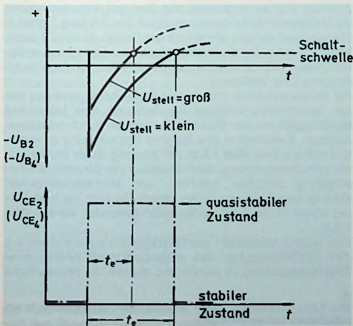
Bild 7.2.3: Einfluß der Stellspannung auf die Einschaltzeit einer monostabilen Kippstufe
