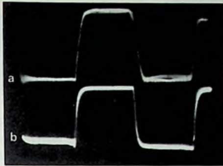
Bild 5: Zeilenoszillogramme des mittleren Bereiches vom Norm-Farbbalken a) ohne, b) mit CTI-Schaltung, gemessen an der B-Kathode
