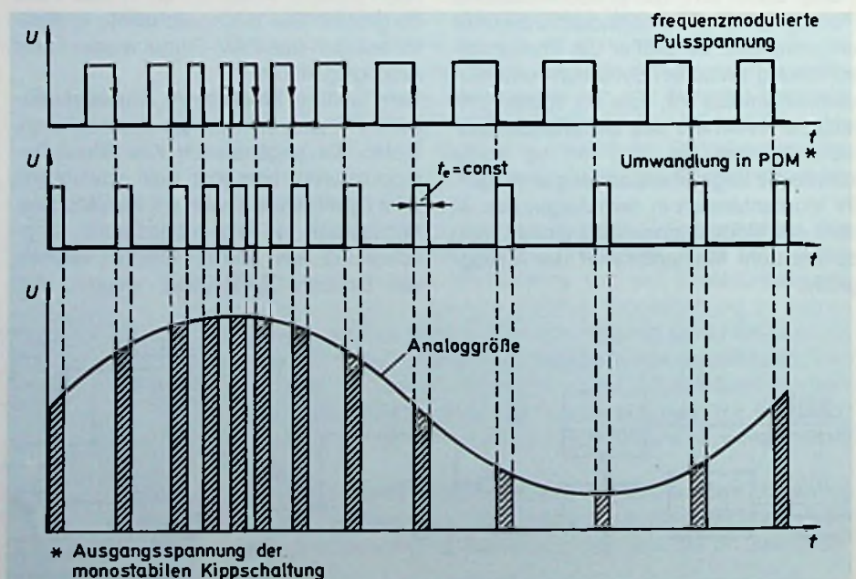
Bild 7.4.2: Zeitlicher Verlauf der Spannungen beim Demodulieren einer frequenzmodulierten Pulsspannung
