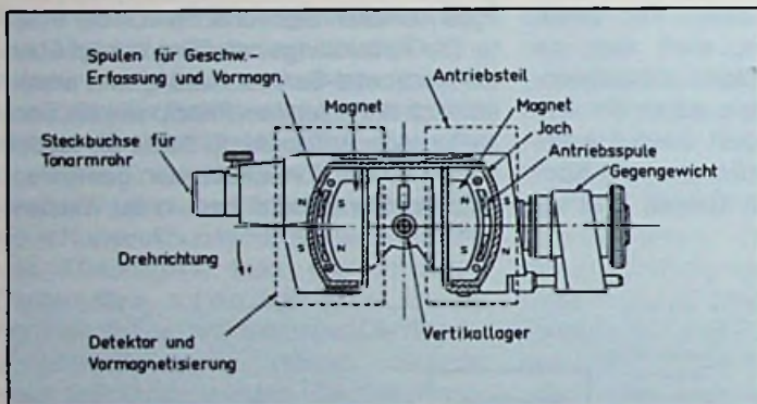
Bild 5: Der mechanische Aufbau des vertikalen Tonarmantriebes
