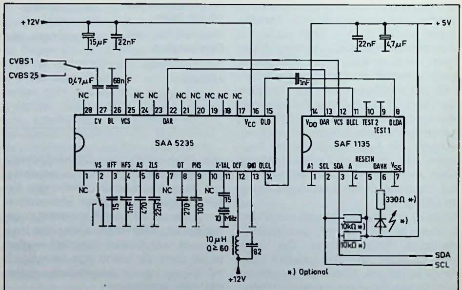
Bild 9: Kompletter 2-Chip VPS-Datenzeilenempfänger der zweiten Generation (s. auch Bild 2) (Bild: Valvo)
