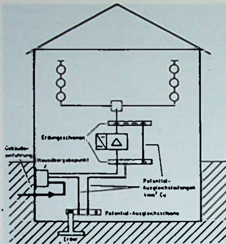
Bild 5: Beispiel für die Hauseinführung eines Antennenkabels und den Anschluß des Hausübergabepunktes sowie Verstärkers an die Potentialausgleichsschiene
