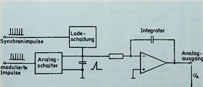
Bild 7.3.6: Prinzipielle Schaltung eines Pulsphasen-Demodulators nach dem Sägezahn-Vergleichsverfahren
