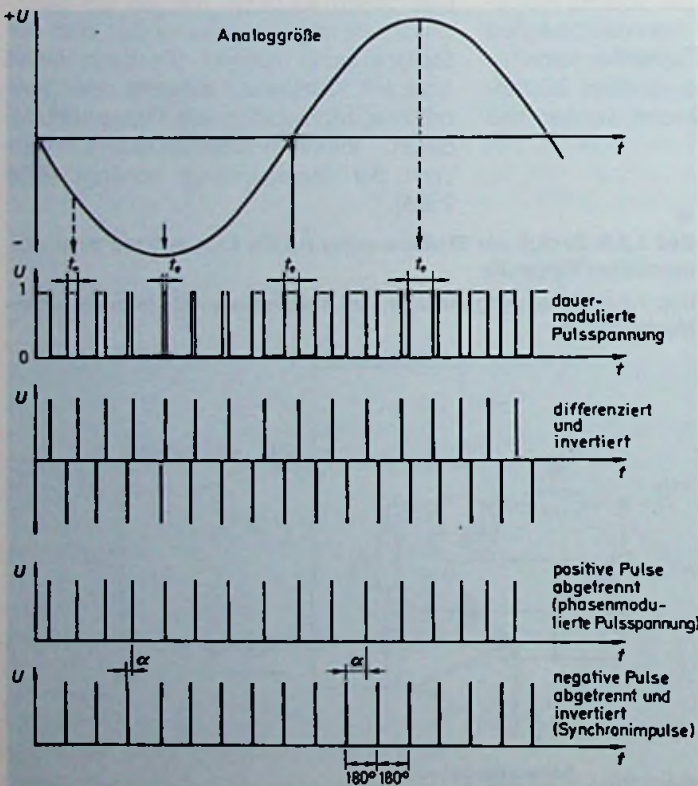
Bild 7.3.1: Umwandlung einer sinusförmigen Analoggröße in ein pulsphasenmoduliertes Signal
