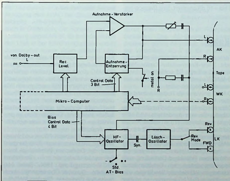
Bild 6: Die Eingriffspunkte des Mikrocomputers in den analogen Aufnahmeverstärker
